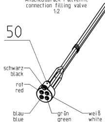
Anschlußstück Füllventil connection filling valve 1:2
