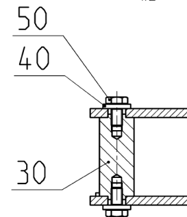
Schnitt/section B-B 1:2
