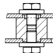
Schnitt/section B-B h= 88mm-149mm ohne oberste Platte und Pos. 25 without highest plate and item 25
