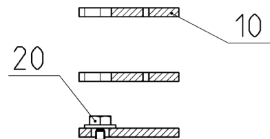
Schnitt/section A-A 1:2
