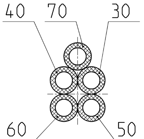
Schnitt/section B-B 5:1
