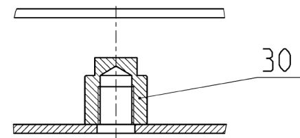
Schnitt/section A-A 1:1
