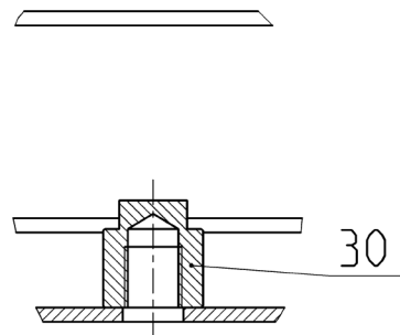
Schnitt/section A-A 1:1
