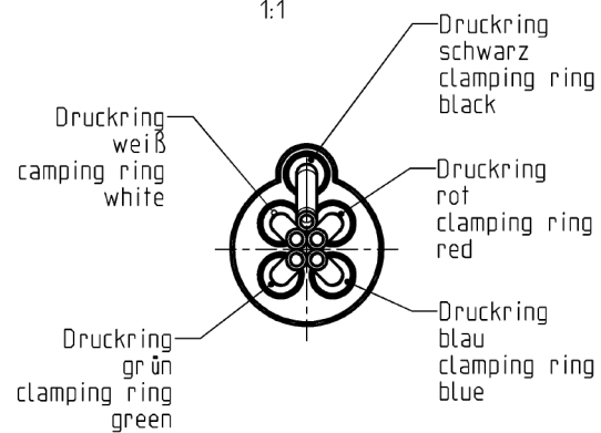
Ansicht/view X 1:1
