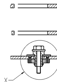
Schnitt/section A-A
