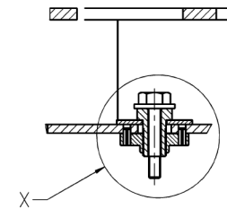
Schnitt/section A-A
